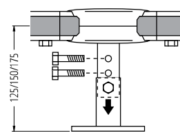
Výškově stavitelná rohová spojka Vario
