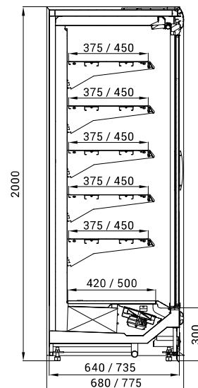
posuvné dveře DP
