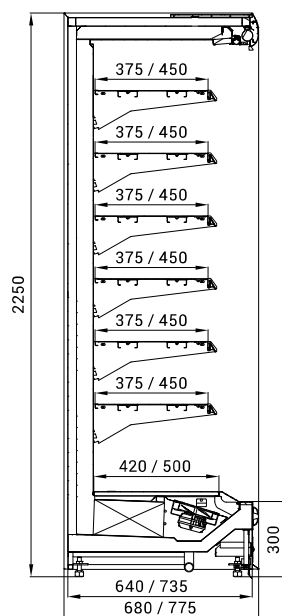
výška 225 cm, 6 polic PLUS
