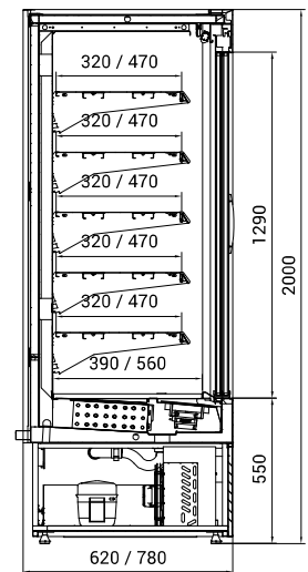
verze s uzamykatelnou roletou RA
